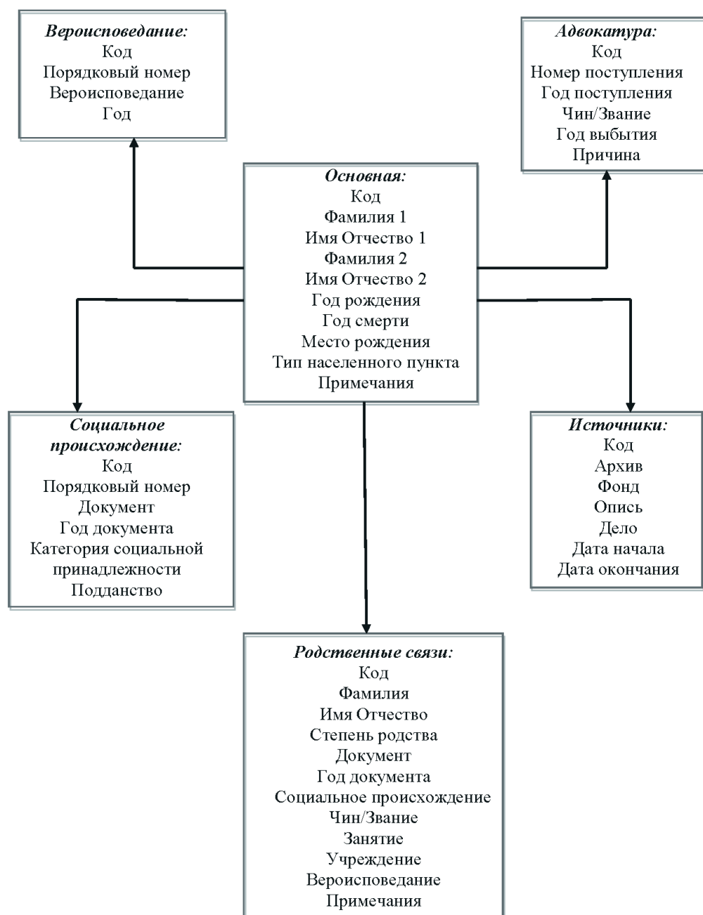
Схема базы данных «Московская корпорация присяжных поверенных (1866–1916 гг.)»
