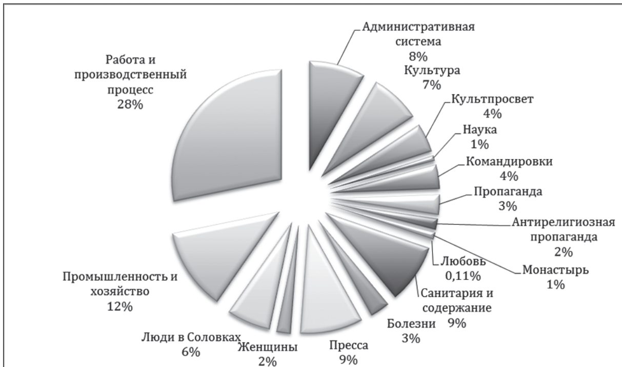
Рис. 2. Частоты встречаемости категорий в 1930 г.
